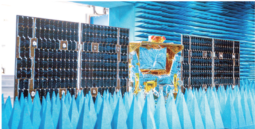
天仪空间协同攻关的“地质一号”卫星。图/天仪空间官网
