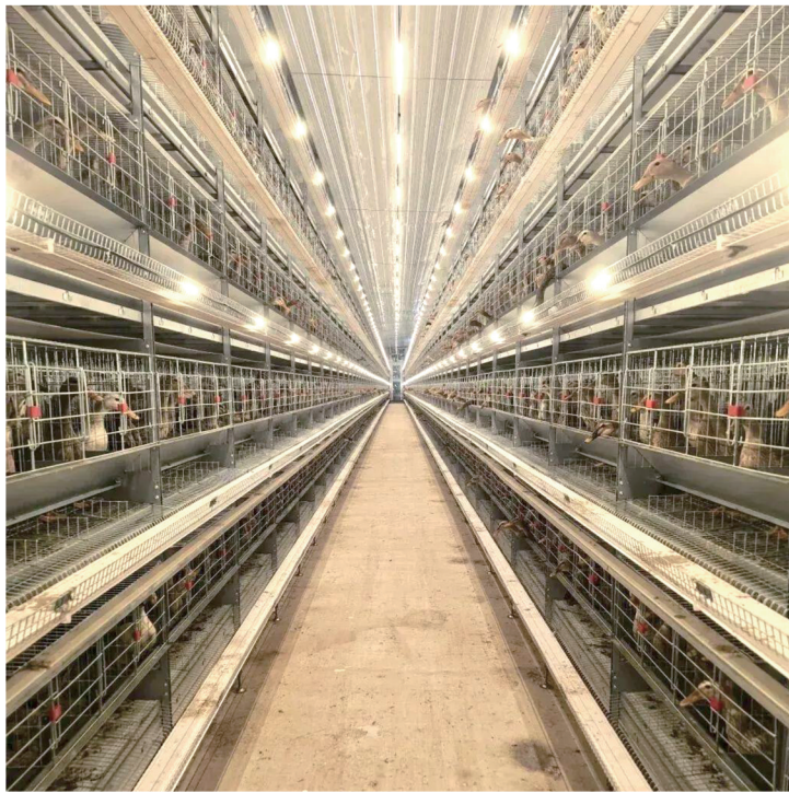
益阳5万羽笼养蛋鸭智能化生产线。图/受访单位提供
